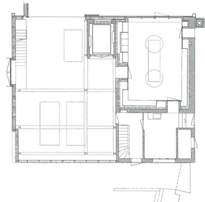
Grundriss Erdgeschoss
